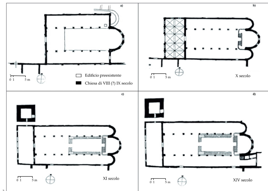
Fig. 12 – Evoluzione nel tempo della chiesa di S. Maria di Pomposa.
